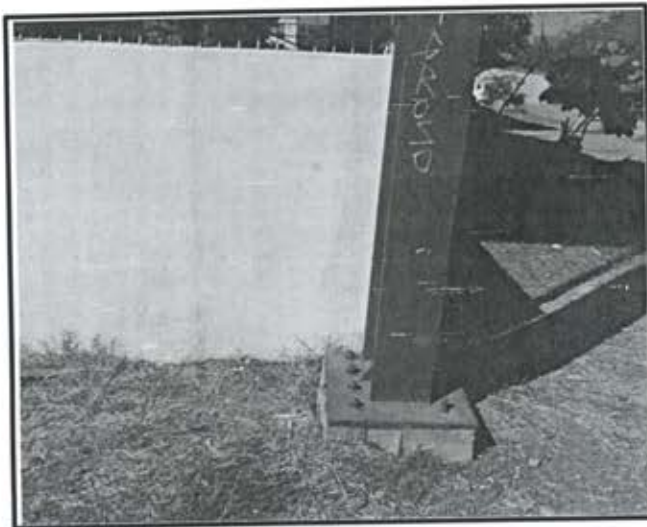
Foto 8. Columna de esquina donde falta tuerca en perno de anclaje.
