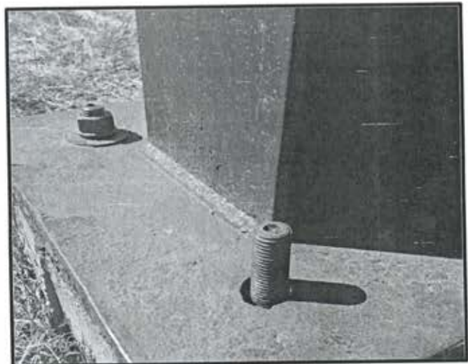
Foto 9. Perno de anclaje sin tuerca
