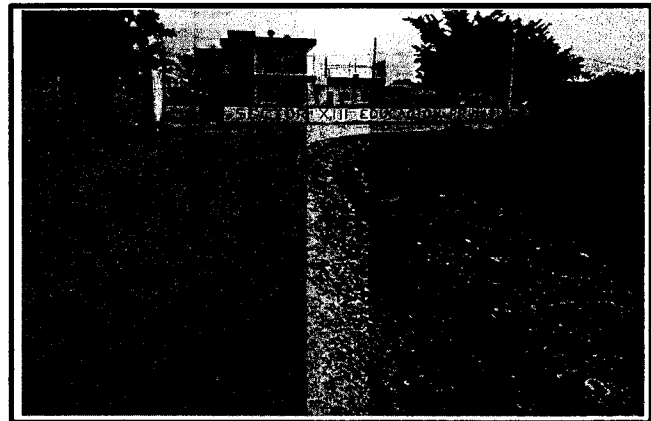
13.- Pavimentacion calle Frenos - colocacion de Riego de sello y sanja para muro de contencion.
