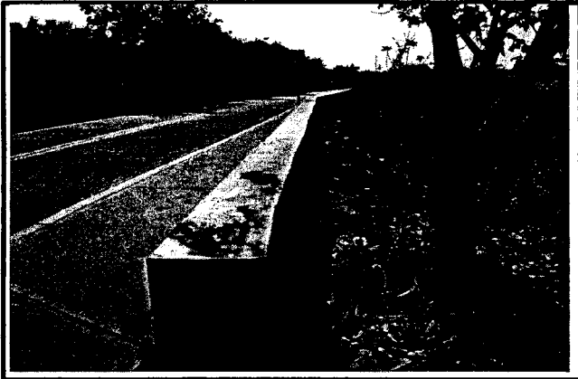
14.- Pavimentacion calle Frenos Concreto Fc 250 kg/cm2
