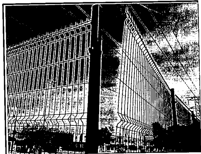
Foto 9. Panel de reja acero sin abrazadera
