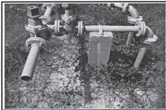
12.- Valvulas y Conexiones para Carcamo Colonia Nuevo Milenio.
