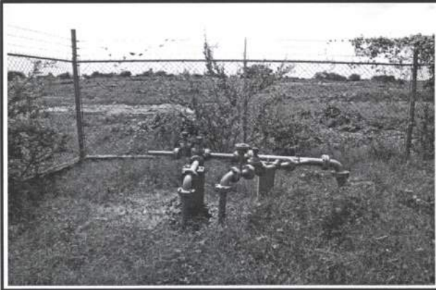
10.- Valvulas y Conexiones para Carcamo Colonia Nuevo Milenio.
